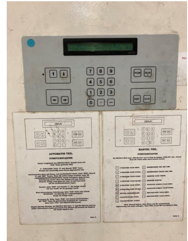
Controle-unit voor het instellen van de palletvoorwaarden
